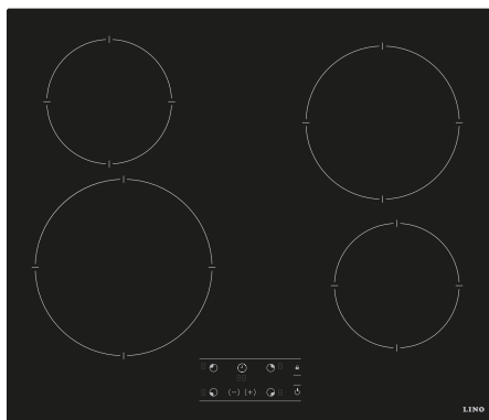
PL3 TCT4 S
