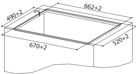
HOO-B GLASS + 2 индукционни плота FCH32 Монтаж за вграждане на едно ниво с работен плот
