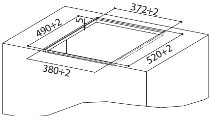
HOO-B GLASS + 1 индукционен плот FCH32 Монтаж за вграждане на едно ниво с работен плот
